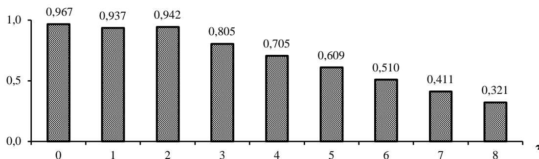
Рис. 1. Кореляційна функція \rho[y_m(t), y_{pg}(t + \tau)] для різних \tau
