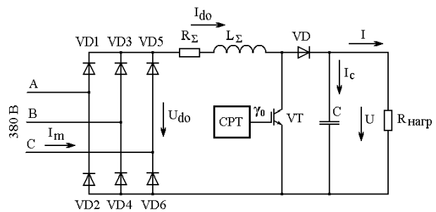
Рис.4. Расчетная схема силовой части АККМ, приведенная к цепи постоянного тока.
