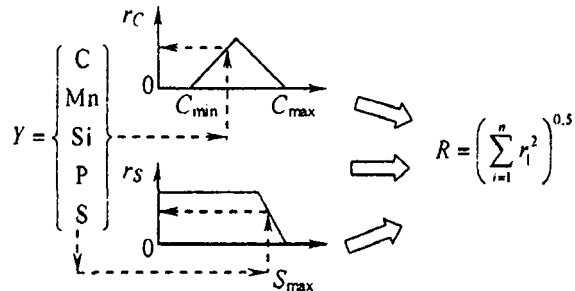
Рис. 1. Формирование обобщенного показателя качества стали
