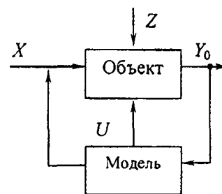
Рис. 2. Схема управления объектом
