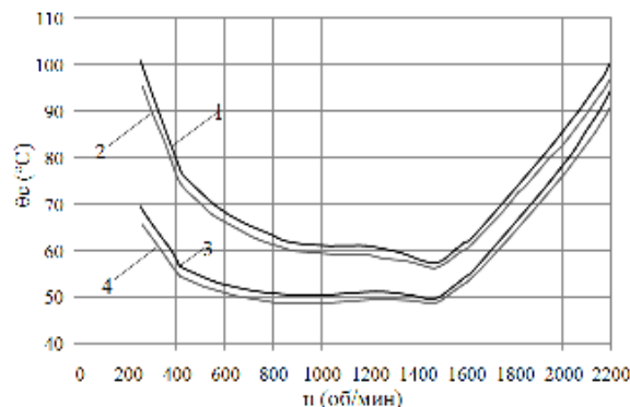
Рис. 1 – Зависимости изменения температуры перегрева обмотки статора: 1 – серийный АД с самохлаждением, 2 – АД с измененным числом параллельных ветвей с самохлаждением, 3 – серийный АД с независимым охлаждением, 4 – АД с измененным числом параллельных ветвей с независимым охлаждением
