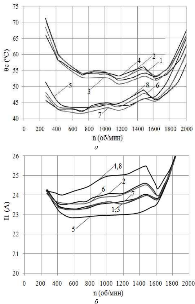
Рис. 2 – Изменение температуры перегрева обмотки статора а, потребляемого тока б в диапазоне регулирования.
