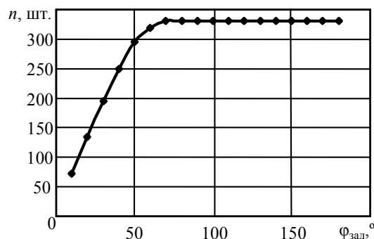
Рис. 4. Зависимость количества твэлов, попадающих в зону облучения коллиматора детектора, от угла облучения коллиматора детектора
