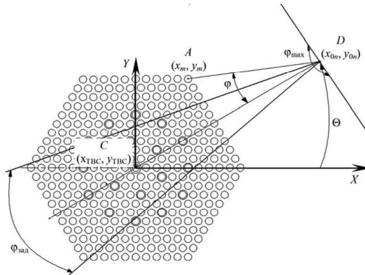
Рис. 1. Картограмма ТВС
