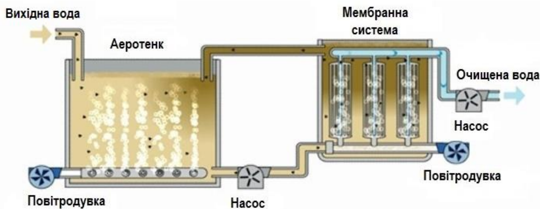
Рис.9.9 – Схема технології мембранного біореактора
