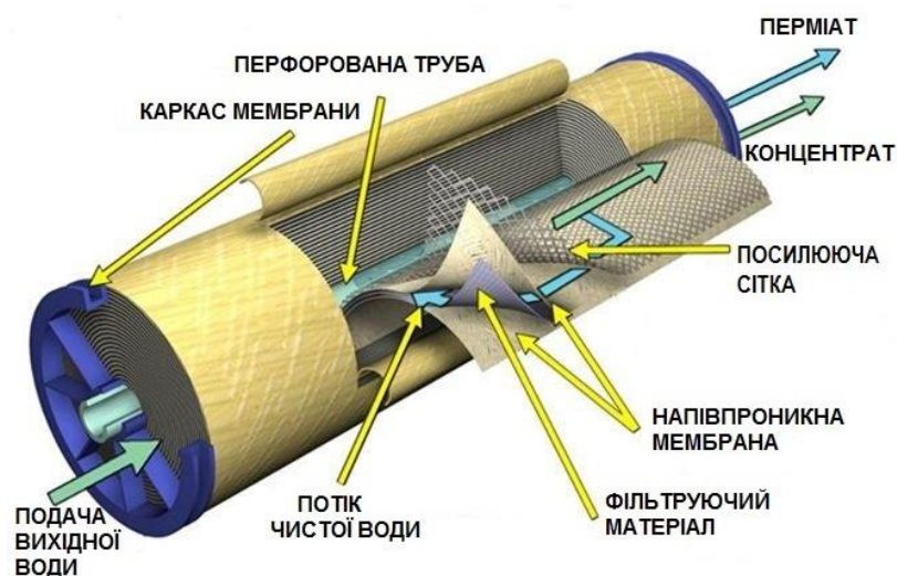
Рис. 7.3 – Рулонний (спіральний) модульний проект
