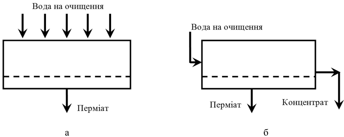
Рис. 7.2 – Схеми напрямку руху потоку води відносно мембрани: а – тупикова; б – тангенціальна
