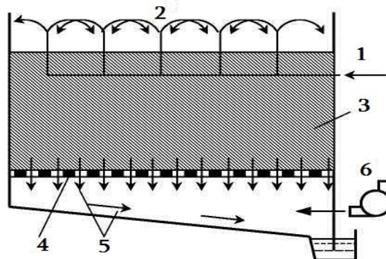
Рис. 9.6 – Схема біофільтра: 1 – подача стічних вод; 2 – водорозподільний пристрій; 3 – фільтрувальне завантаження; 4 – дренажний пристрій; 5 – очищена стічна вода; 6 – пристрій повітря розподільний
