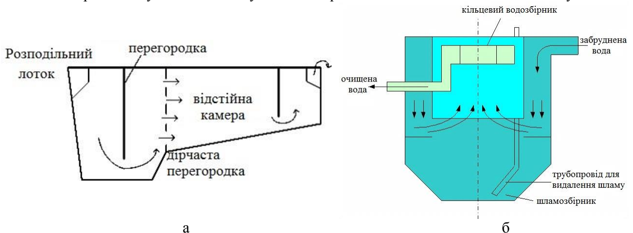
Рис. 4.1 – Схеми відстійників
