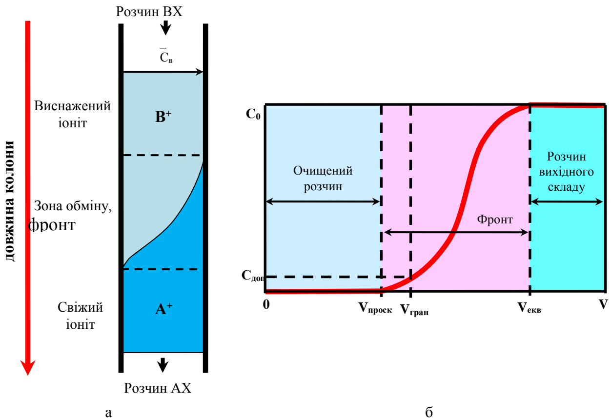
Рис. 6.3 – Динаміка іонного обміну: а – схема іонообмінного процесу в колоні; б – вихідна крива іонного обміну
