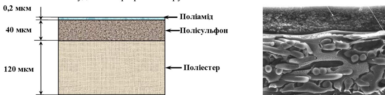
Рис. 7.7 – Структура композитного мембранного полотна та його фотографія
