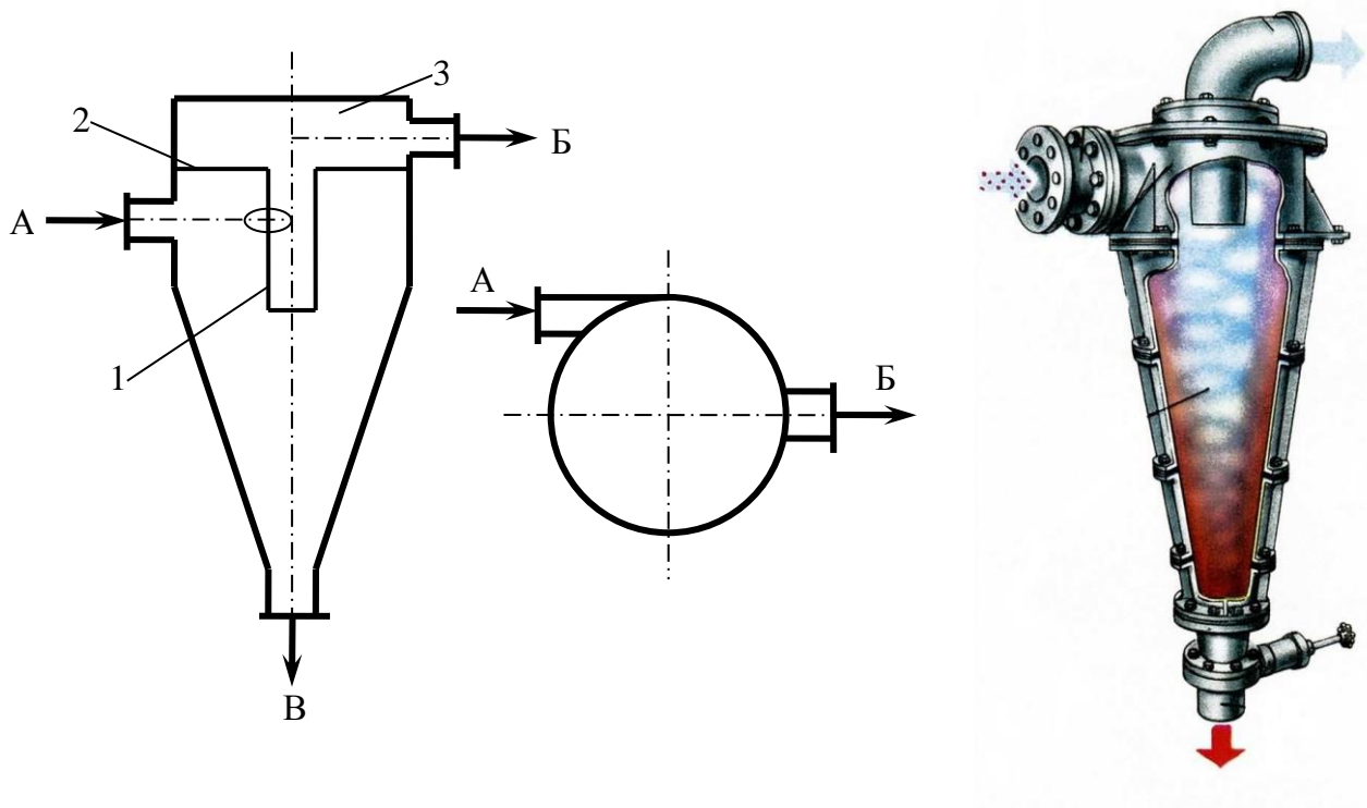
Рис. 4.6 – Схема гідроциклону
