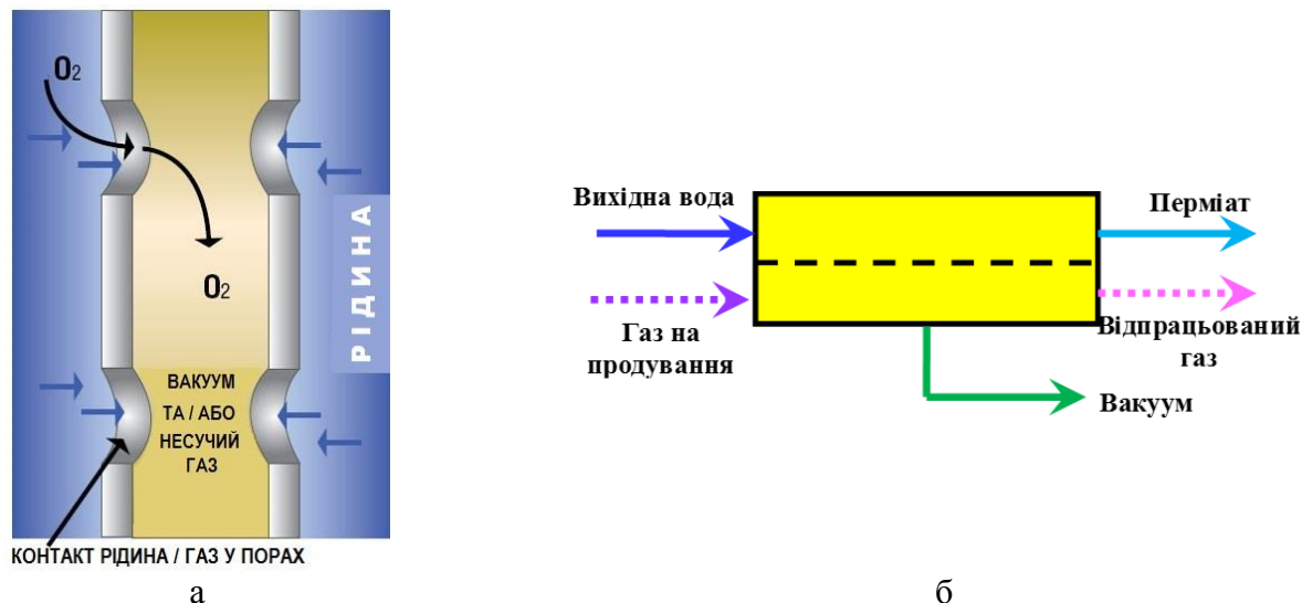
Рис. 7.11 – Принцип роботи мембранного порожнистолоконтурного елемента (а) та схема організації процесу мембранної дегазації (б)
