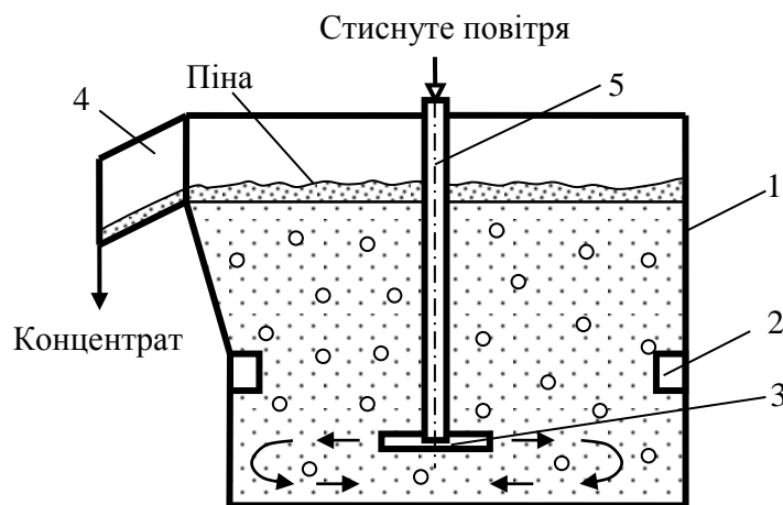
Рис. 4.4 – Принципова схема пневмомеханічної флотомашини: 1 – камера (корпус); 2 – стабілізатори; 3 – імпелер; 4 – переливний поріг; 5 – порожнистий вал
