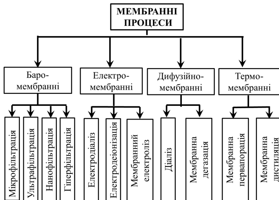
Рис. 7.1 – Класифікація мембранних процесів
