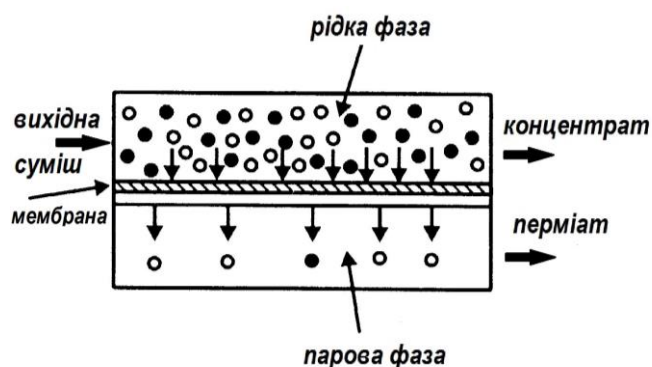
Рис. 7.13 – Принципова схема мембранної первапорації
