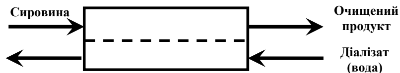
Рис. 7.10 – Принципова схема діалізу
