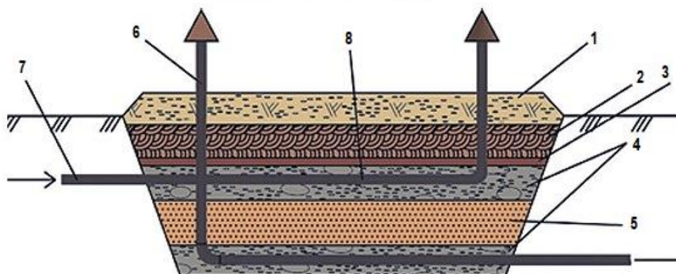
Рис. 9.3 – Схема піщано-гравійного фільтру: 1 – утеплюча засипка; 2 – глиняний замок; 3 – гідроізоляція; 4 – зона зрошення (щебінь); 5 – пісок; 6 – вентиляційний стояк; 7 – підвідний трубопровід; 8 – зрошувальні труби
