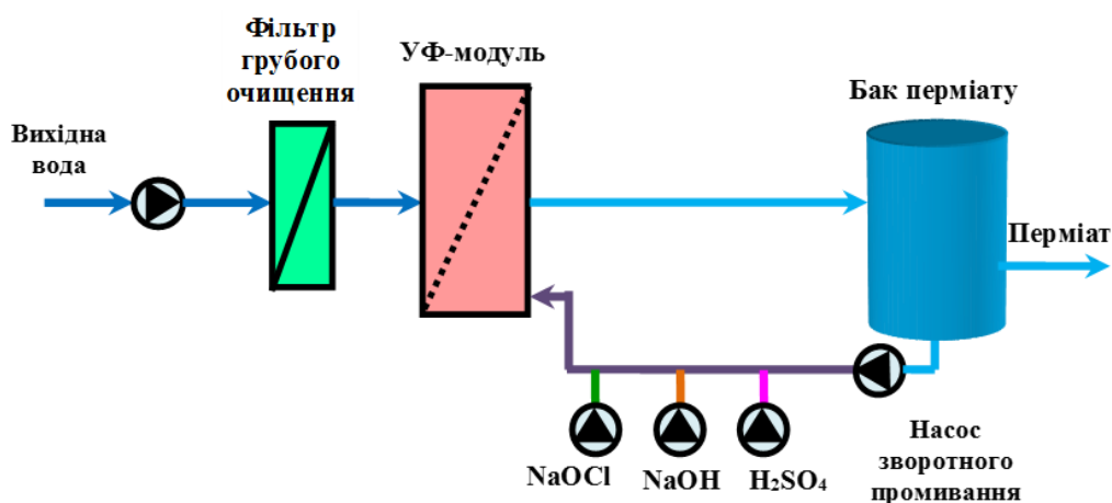
Рис. 7.4 – Принципова технологічна схема ультрафільтрації, яка працює у режимі тупикового фільтрування зі зворотним промиванням фільтратом
