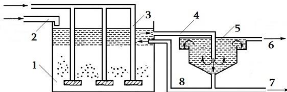
Рис. 9.7 – Схема роботи аеротенка: 1 – аеротенк, 2 – подача стічної води, 3 – подача повітря, 4 – активний мул, 5 – відстійник, 6 – очищений стік, 7 – надлишковий мул, 8 – поворотний мул
