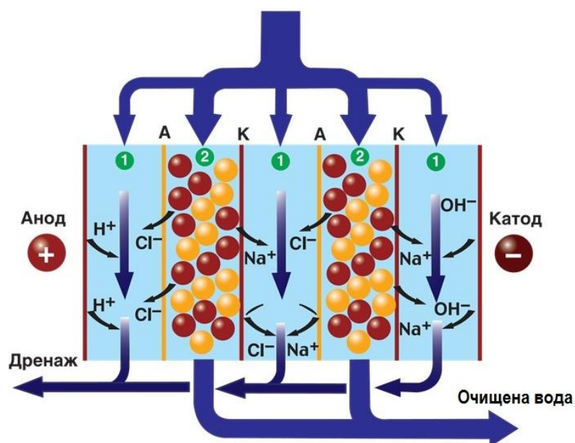
Рис. 7.14 – Схема електродеіонізаційної установки
