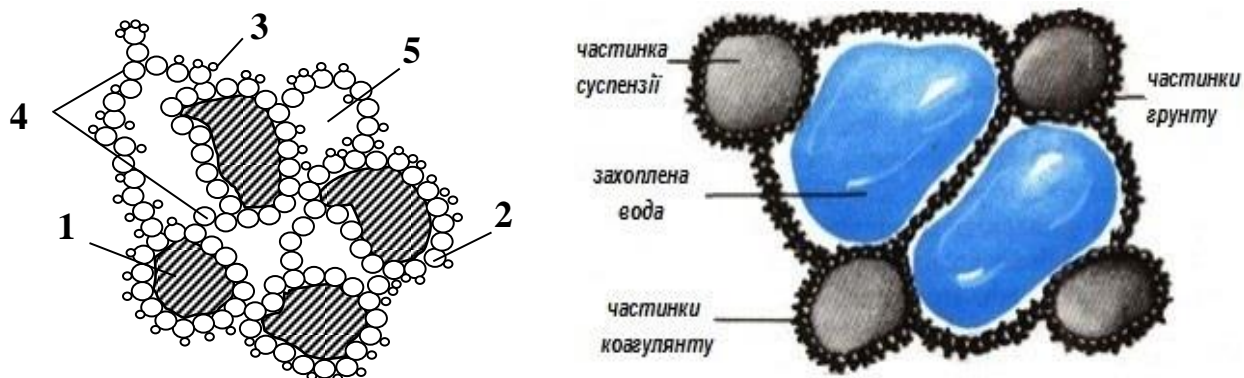
Рис. 4.5 – Схема утворення флокул
