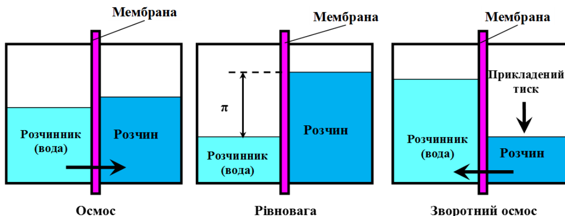
Рис. 7.5 – Схема процесів осмосу та зворотного осмосу
