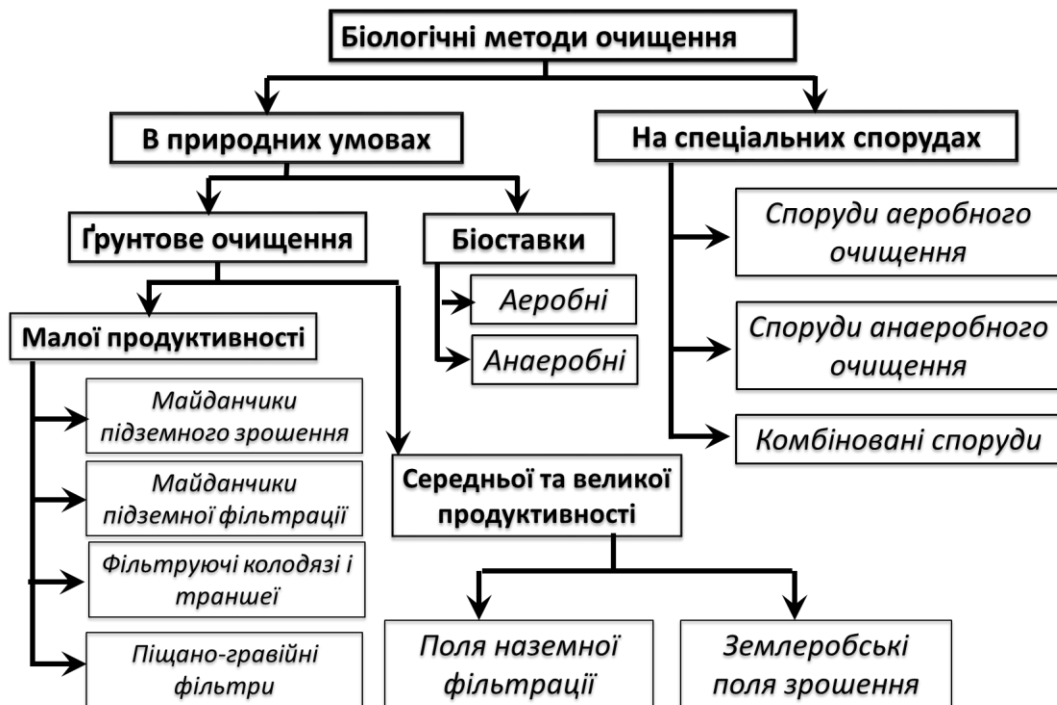
Рис. 9.1 – Класифікація споруд біологічного очищення
