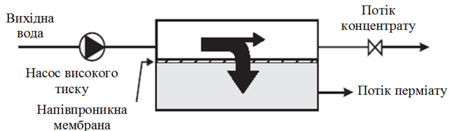
Рис. 7.8 – Принципова схема системи зворотного осмосу і нанофільтрації
