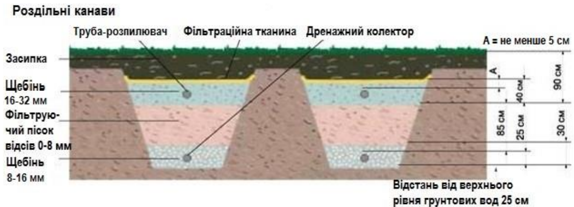
Рис. 9.2 – Схема поля підземної фільтрації з роздільними каналами
