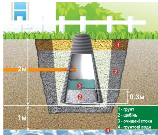
Рис. 9.5 – Схема фільтруючого колодязя
