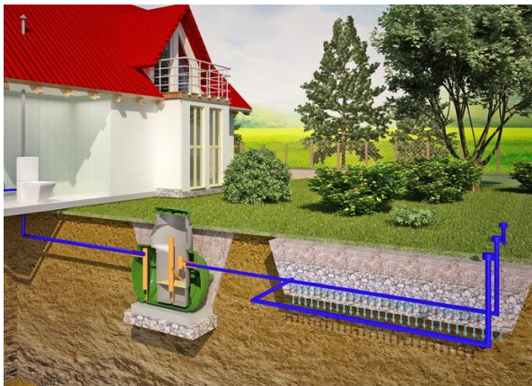
Рис. 9.4 – Схема фільтруючої траншеї
