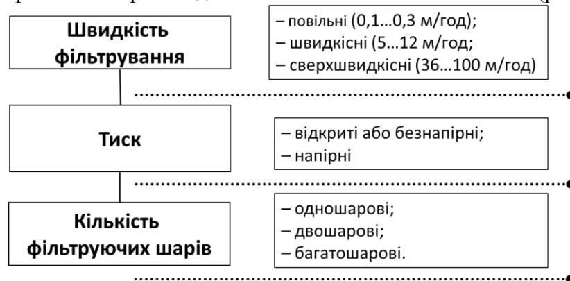
Рис. 4.3 – Класифікація фільтрів із зернистим шаром
