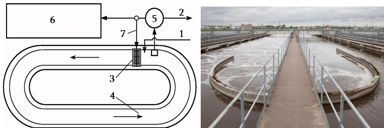
Рис. 9.8 – Схема циркуляційного окиснювального каналу
