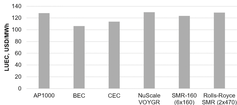
Рисунок 3 – Результати розрахунку LUEC для базового сценарію
