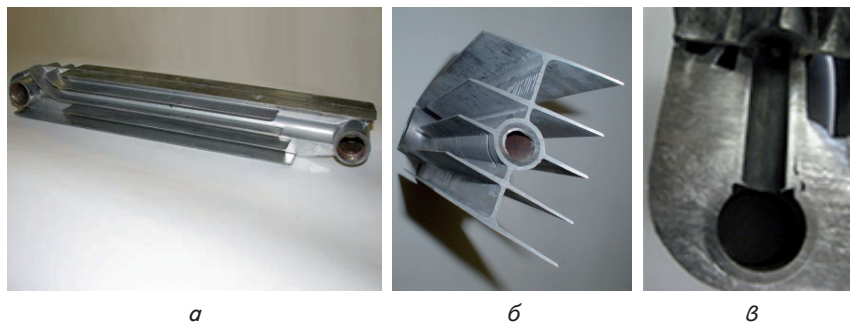
Рис. 4. Изображения биметаллической отливки, изготовленной в Одесском ГП: а — секция радиатора; б — годная деталь в разрезе; в — вид бракованной детали
