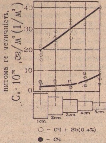
Рисунок 6 - Залежності питомої герметичності сірого чавуну й чавуну, легованого сурмію, від товщини стінки технологічної проби
