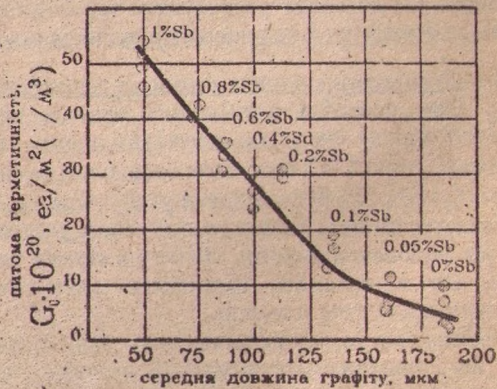
Рисунк 5 - Залежність питомої герметичності сурм'янистого чавуну від довжини графітового включення
