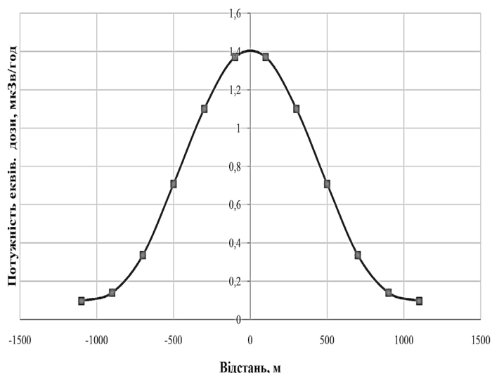
Рис. 2. Розподіл потужності дози в напрямку, перпендикулярному осі факела викиду, при МПА на ХАЕС
