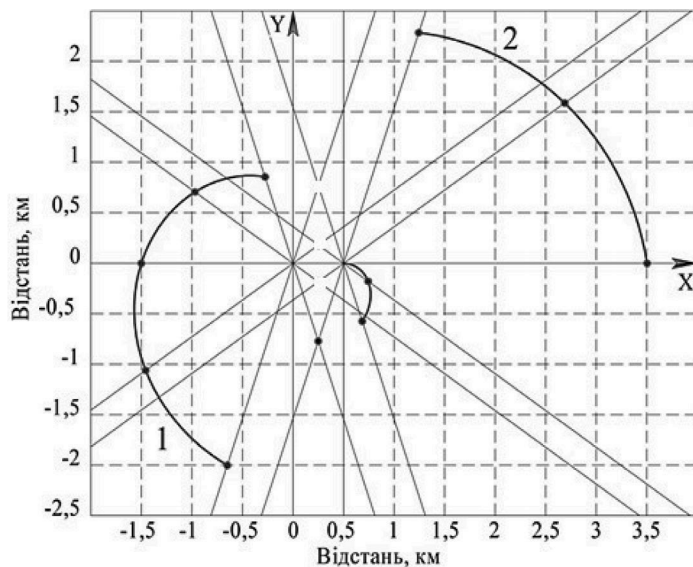
Рис. 5. Схема розміщення \gamma -датчиків АСКРО у СЗЗ для двох енергоблоків ХАЕС
