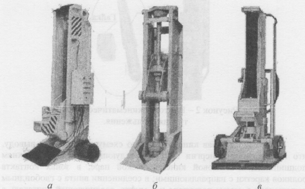
Рисунок 1 – Винтовые домкраты различных производителей: а) ПАО Одесский машиностроительный завод «Красная гвардия» (Украина); б) Кубаньжелдормаш (Россия); в) Whiting corporation, Monee (Illinois, USA).
