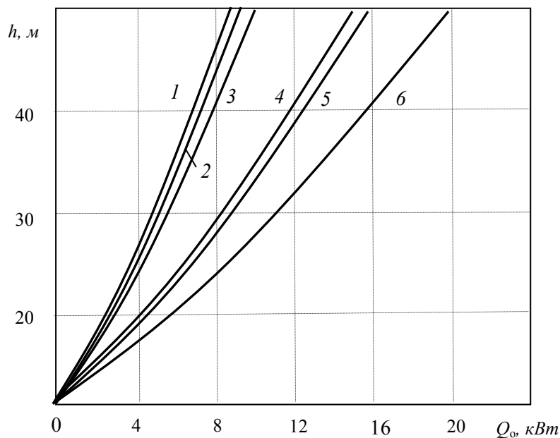
Рис.2. Зависимость оптимальной глубины зонда от расчетной отопительной нагрузки потребителя, температуропроводности грунта и широты местности:
