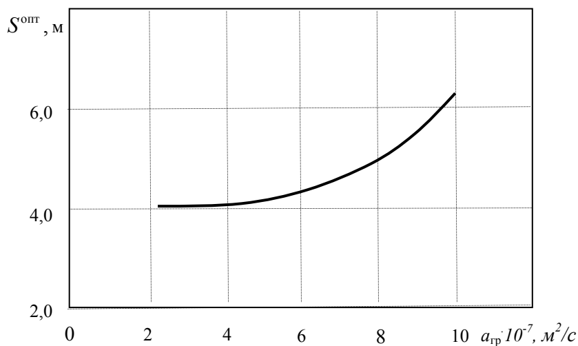
Рис.1. Зависимость оптимального шага зондов от температуропроводности грунта a_{\text{гр}}
