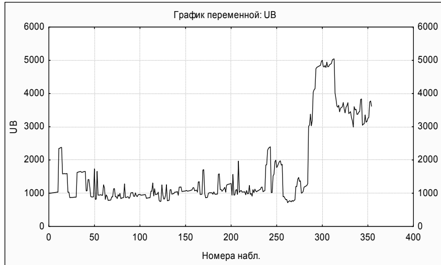
Рисунок 2 – Щоденна динаміка індексу українських облігацій (UB) з 2.01.2013 р. по 30.05.2014 р.
