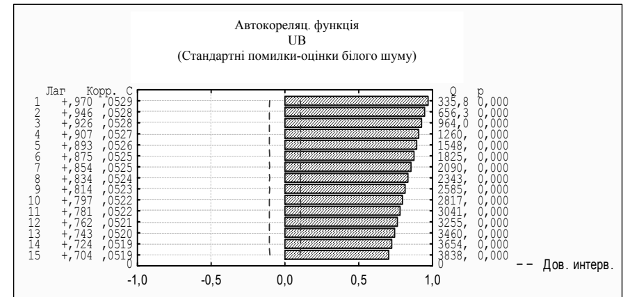
Рисунок 3 – Графік та значення АКФ динаміки UB_t
