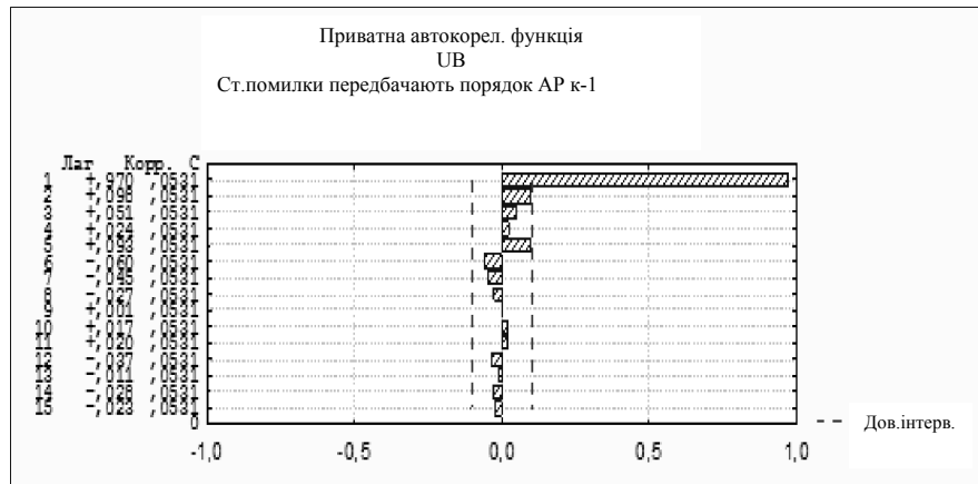
Рисунок 4 – Графік та значення ЧАКФ динаміки UB_t
