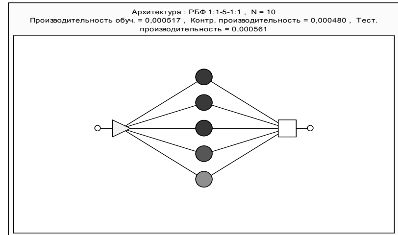
Рисунок 6 – Модель тришарового перцептрону із одним прихованим шаром
