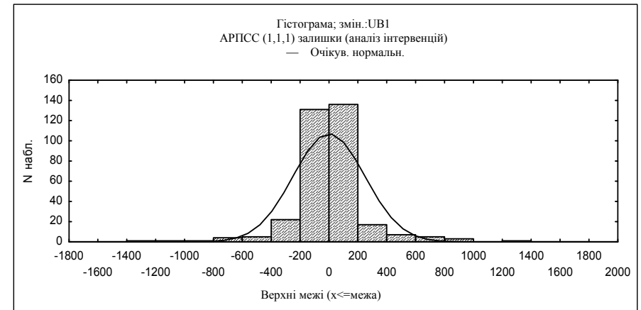
Рисунок 5 – Графік залишків при моделюванні динаміки та порівняння їх із нормальним розподілом
