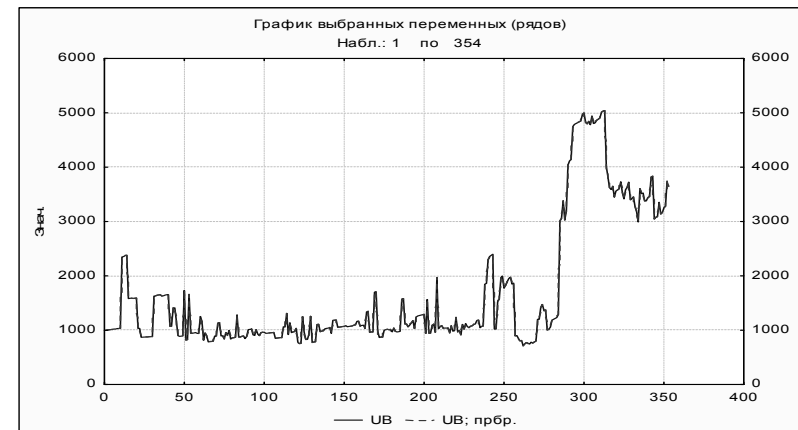
Рисунок 7 – Графіки рядів динаміки (UB– вихідний та UB; прбр. – оптимальна модель).
