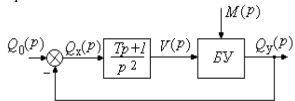
Рис.4. Упрощенная структурная схема системы
