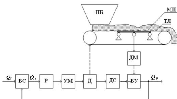
Рис. 1. Упрощенная функциональная схема системы управления непрерывного ленточного дозатора
