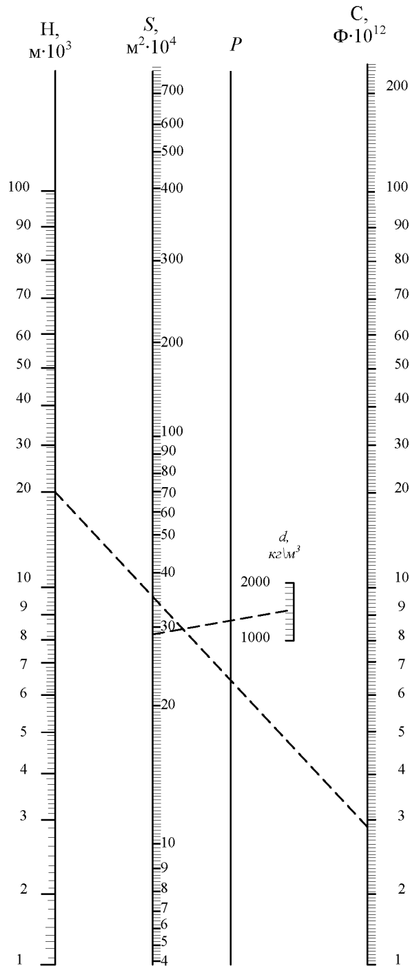
Рис. 3. Номограмма для расчета плотности оболочковых форм
