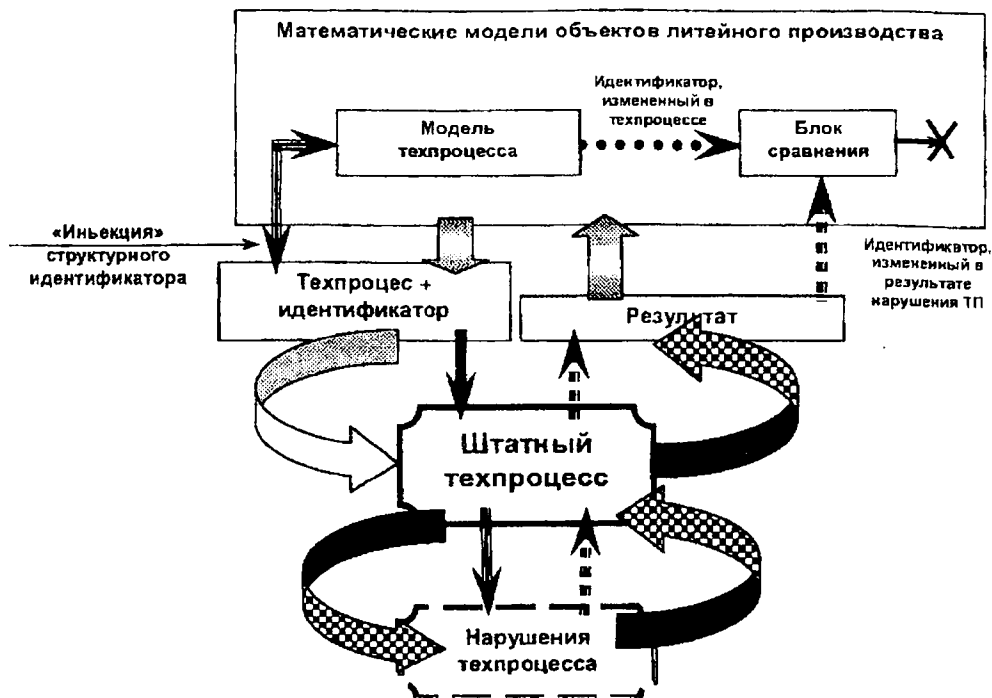
Рисунок 1 – Схема метода структурных идентификаторов
