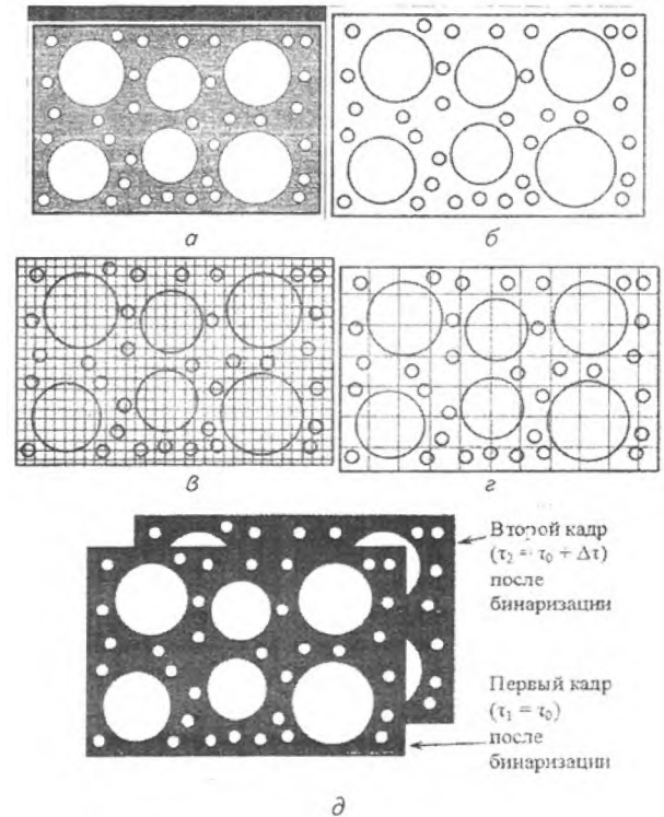
Рис. 3. Схемы этапов свертки поверхности теплообмена: а – томограмма (сечение); б – выделенные границы в сечении; в – к расчету хаусдорфовой размерности границ в сечении; г – к свертке с помощью принципа сжимающих отображений; д – два последовательных кадра после бинаризации, готовые к свертке с помощью параболического преобразования
