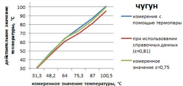
Рисунок 2 – Влияние коэффициента излучательной способности на точность бесконтактного метода измерения температуры стали и чугуна
