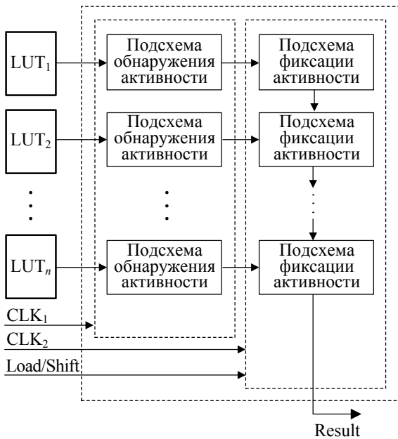
Рис. 1. Обобщенная структура схемы регистрации активности блоков LUT
