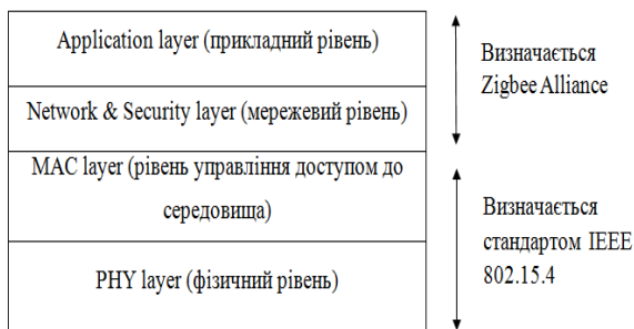
Рис.1. Архітектура безпроводних сенсорних мереж IEEE 802.15.4/Zigbee
