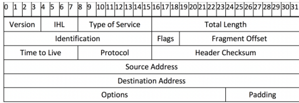
Fig. 1. Internet header.
