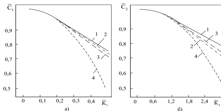
Рис. 2. Залежність фазової швидкості «швидкої» (а) та «повільної» (б) мод хвильового числа:
