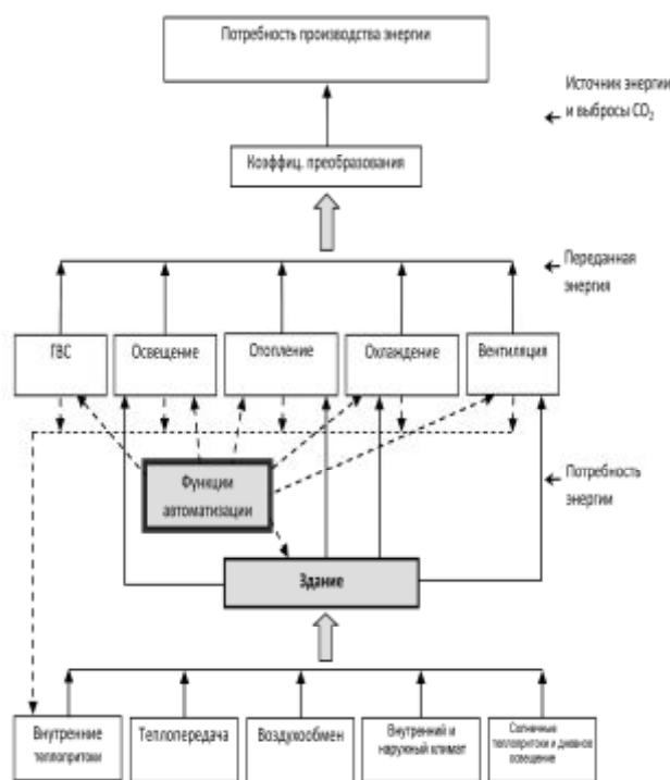
Рис. 8. Отдельные этапы расчетов и взаимосвязь энергетических потоков
