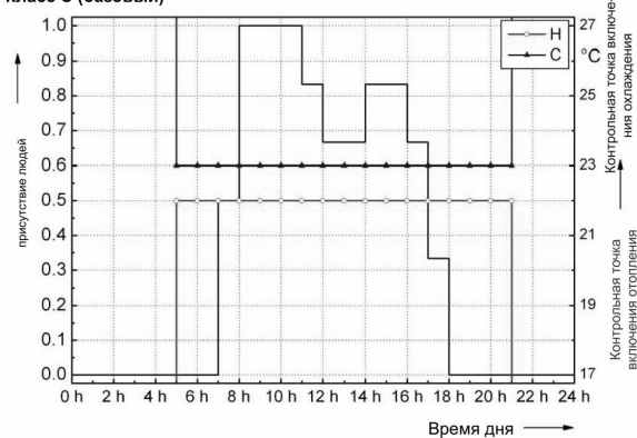
Рис. 4. Эксплуатационный профиль офисного здания. Класс C
