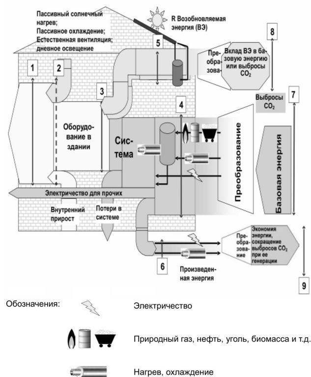
Рис. 7. Модель теплоток для поддержания заданной температуры в помещении
