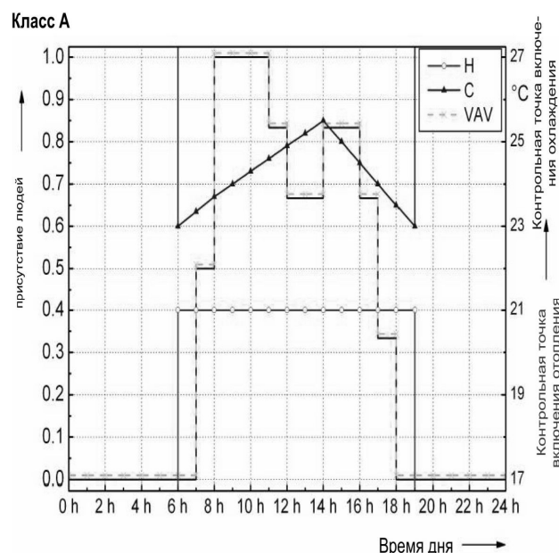
Рис. 6. Эксплуатационный профиль офисного здания. Класс А
