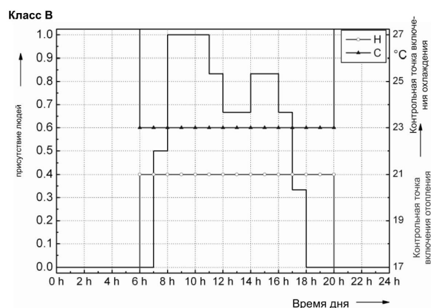
Рис. 5. Эксплуатационный профиль офисного здания. Класс В
